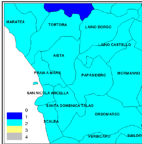
Figura 1 – Classificazione sismica
